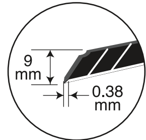
S-Blades
